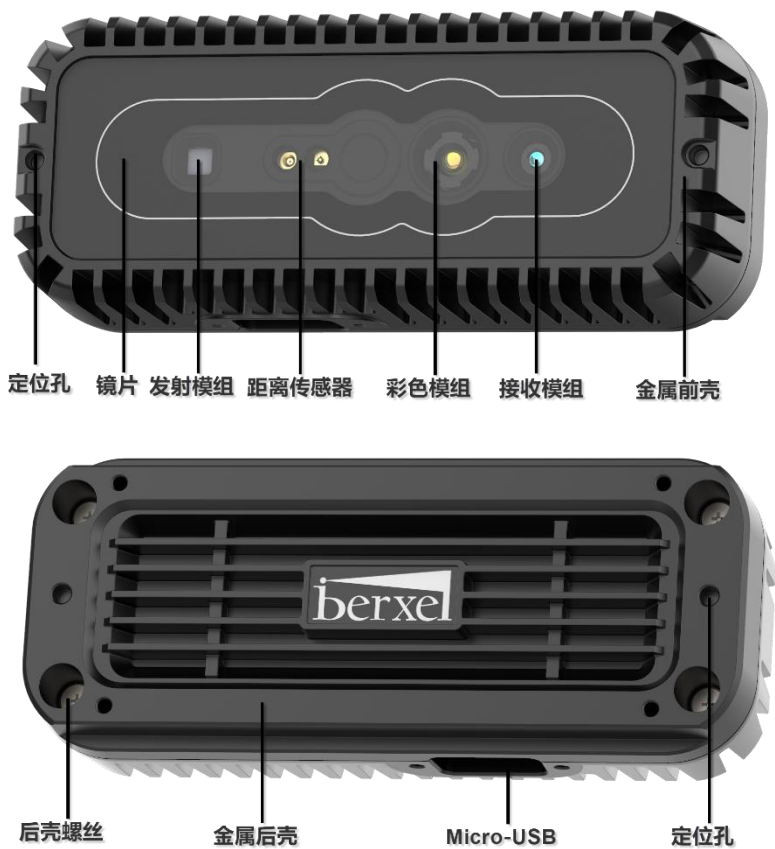
图 2 组件示意图
