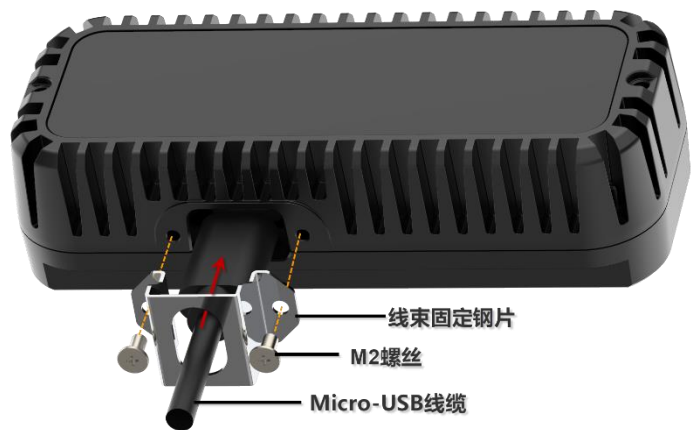
图 5 线缆固定示意图
